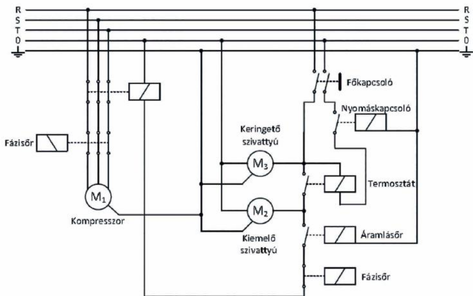
Hőszivattyú elektromos rajza
