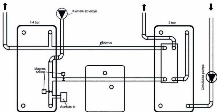
Hőszivattyú kapcsolási rajza
